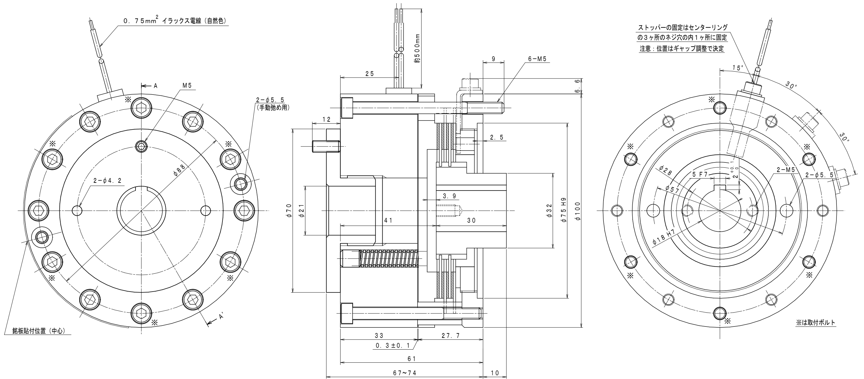
A-A' 断面
