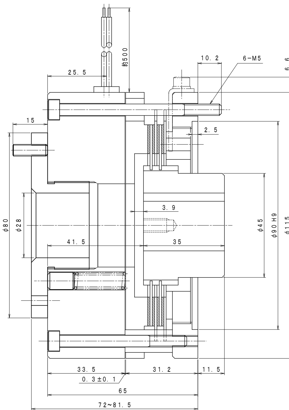
A-A' 断面
