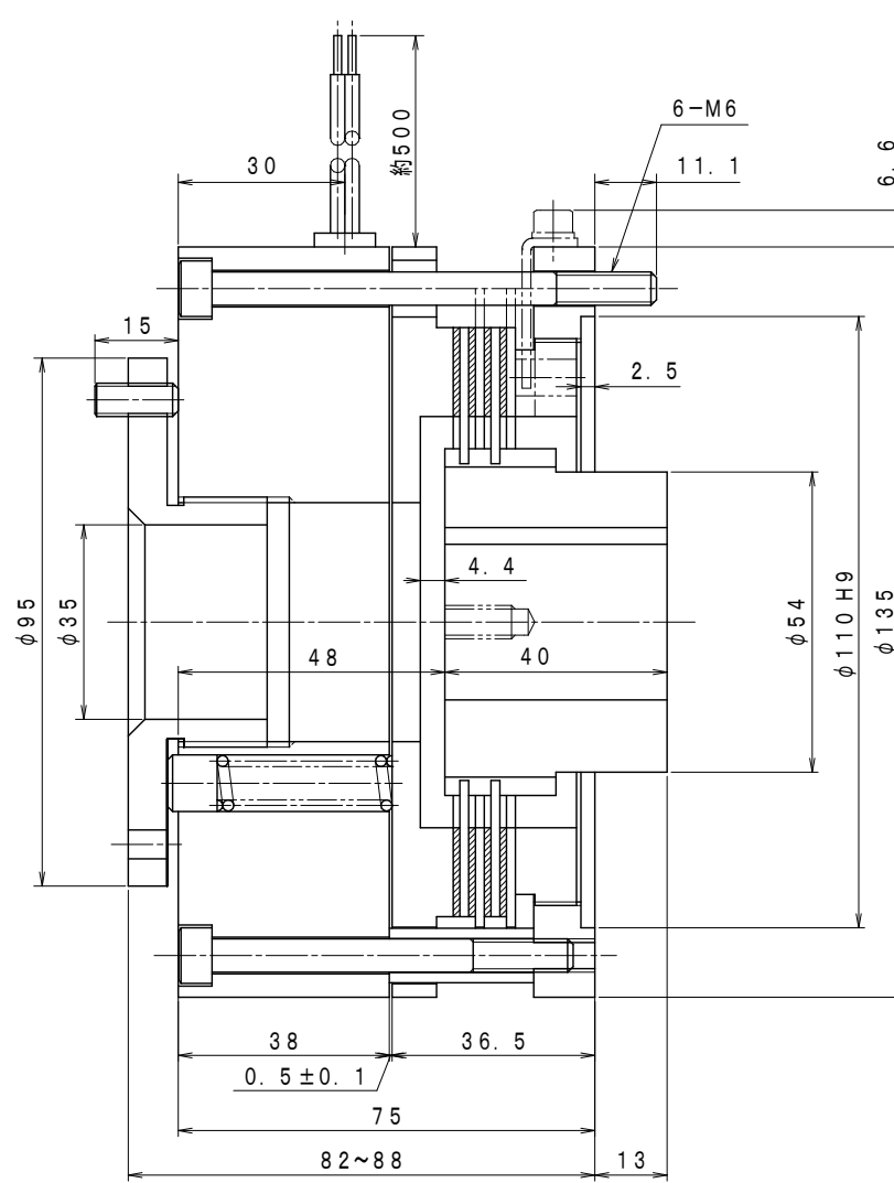
A-A' 断面
