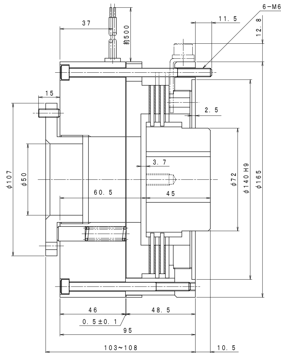
A-A' 断面
