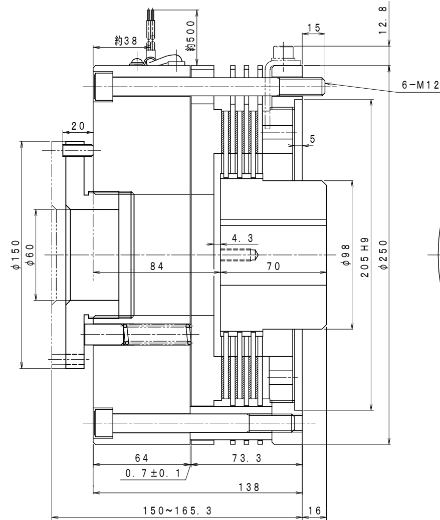
A-A' 断面
