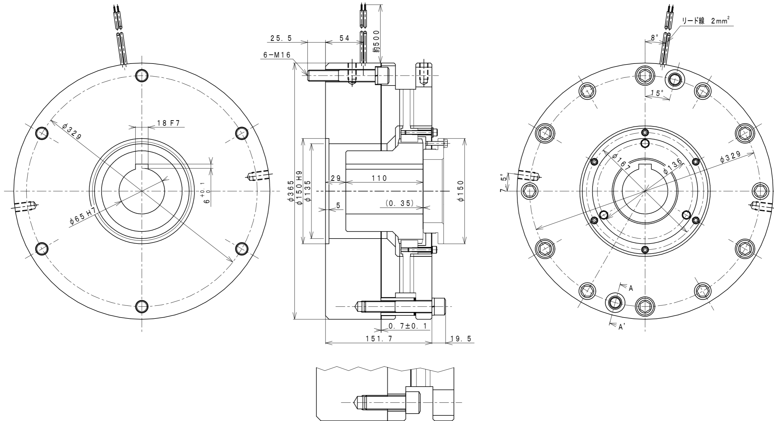
A-A' 断面 (手動解放時)
